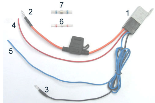
Bild 2 Versorgungs-Satz
